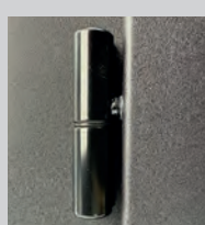
Fiches laquées Ø13x60 réglables à vis invisibles et bagues Téflon anti-usure sans rupture de joint
