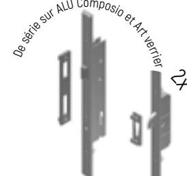
Serrure à crochets SR 3 points à relever - avec 1 pêne central et 2 crochets
