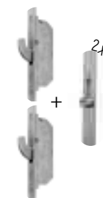
Serrure automatique SAC 5 points à crochets : - avec 2 crochets, 1 pêne central à déclenchement automatique
