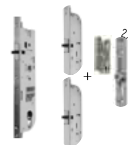
Serrure automatique SAM 5 points ouverture à la clé : - avec 3 pènes - 2 galets champignon + gâches antiécartement - enclenchement automatique des 3 pènes - verrouillage des 2 galets par manoeuvre à la clé - Nécessaire si poignée de tirage
