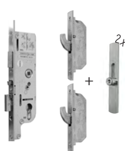
Serrure automatique SAC 5 points à crochets : avec 2 crochets, 1 pêne central à déclenchement automatique
