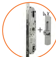
Serrure à relevage 5 points (SR) avec 4 rouleaux + pêne demi-tour
