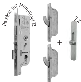
Serrure automatique SAC 5 points à crochets : avec 2 crochets, 1 pêne central à déclenchement automatique
