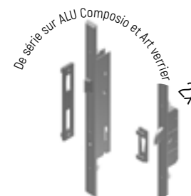
Serrure à crochets SR 3 points à relever - avec 1 pêne central et 2 crochets
