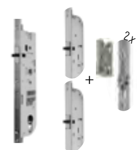
Serrure automatique SAM 5 points «à enclenchement soft» : - avec 3 pénes - 2 galets champignon + gâches antiécartement - enclenchement automatique des 3 pénes en douceur - verrouillage des 2 galets par manoeuvre à la clé
