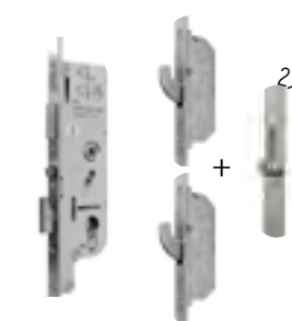
Serrure automatique SAC 5 points à crochets «sécurité +» : - avec 2 crochets, 1 pêne central et 2 rouleaux à déclenchement automatique
