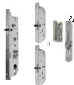
Serrure automatique SAM 5 points «à enclenchement soft»: - avec 3 pènes - 2 galets champignon + gâches antiécartement - enclenchement automatique des 3 pènes en douceur - verrouillage des 2 galets par manœuvre à la clé
